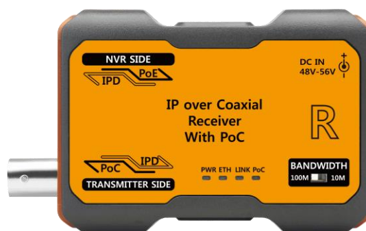
SC-IPR07P (1CH 受信機)
