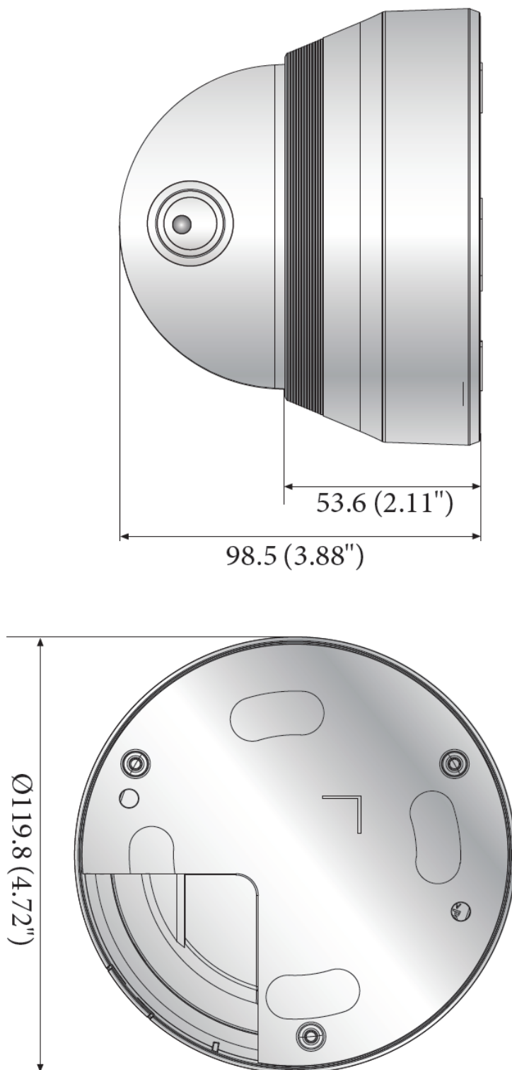
寸法図(mm)
