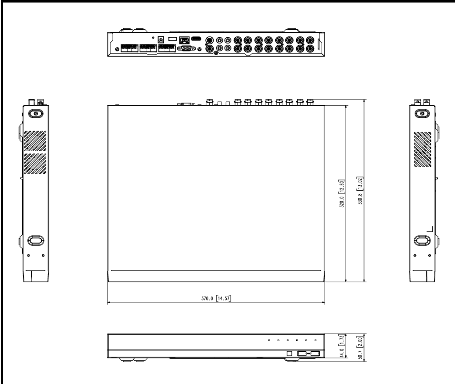
寸法図(mm)
