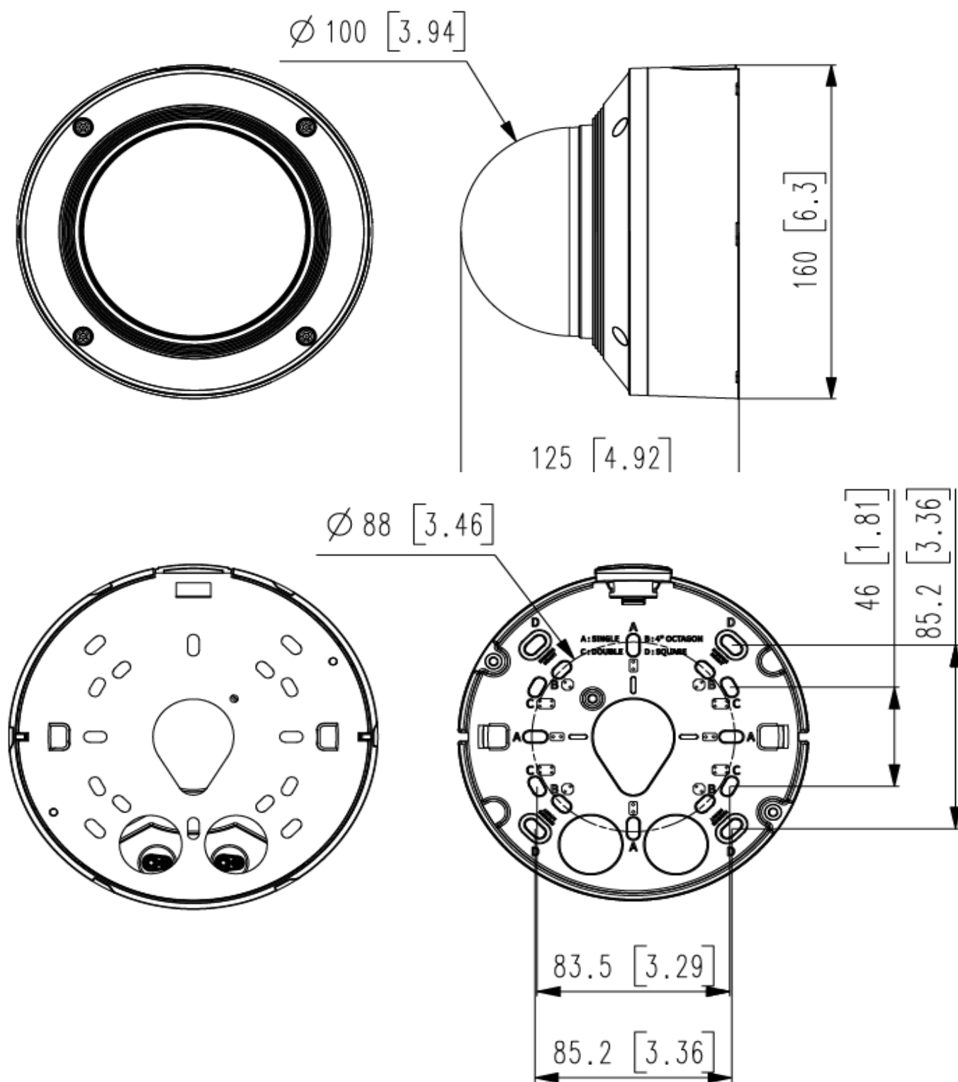
寸法図(mm)
