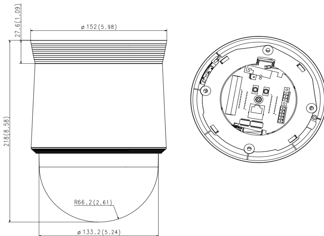
寸法図(mm)
