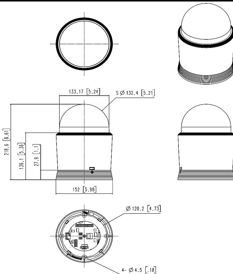
寸法図(mm)
