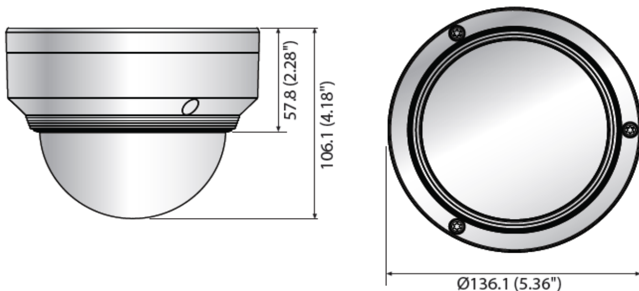
寸法図(mm)
