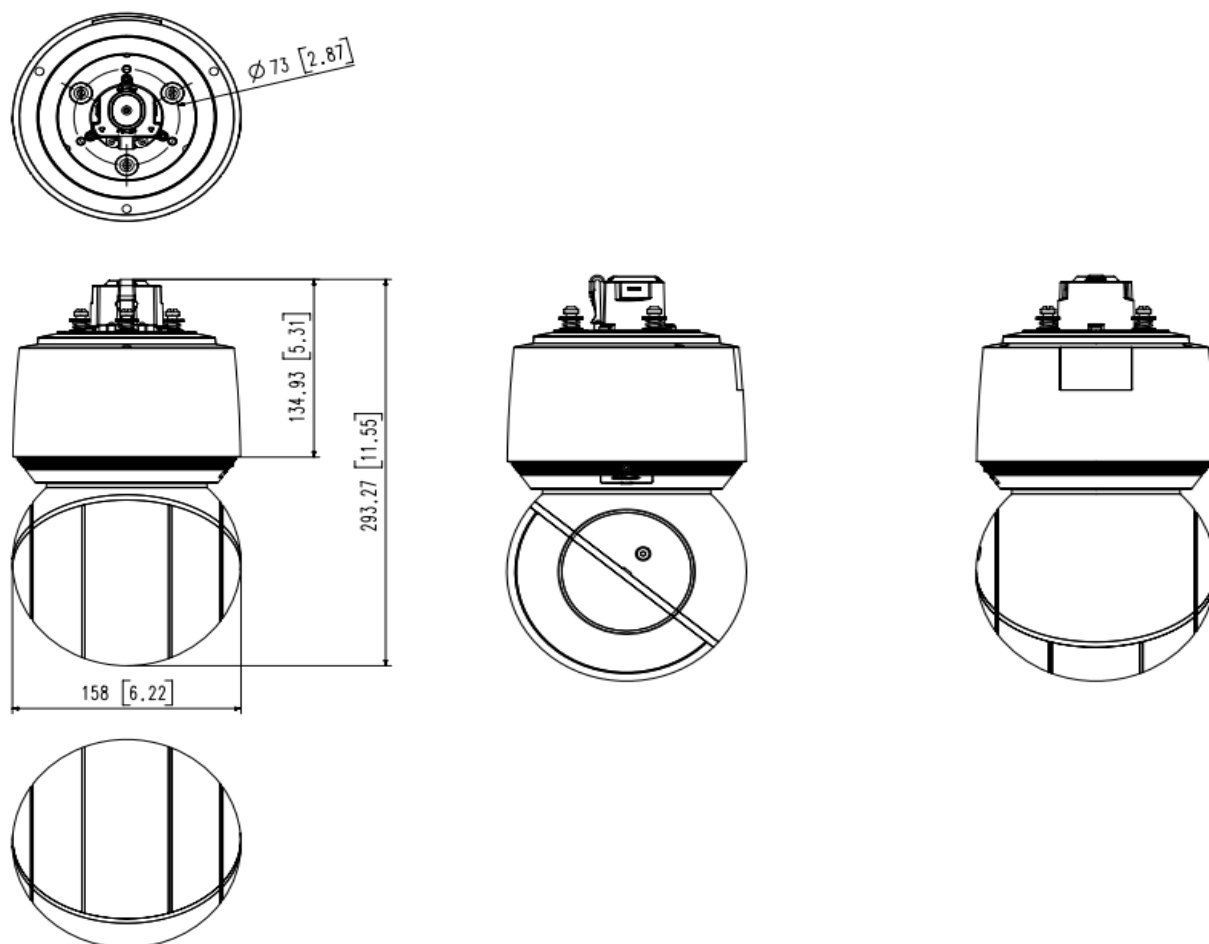
寸法図(mm)
