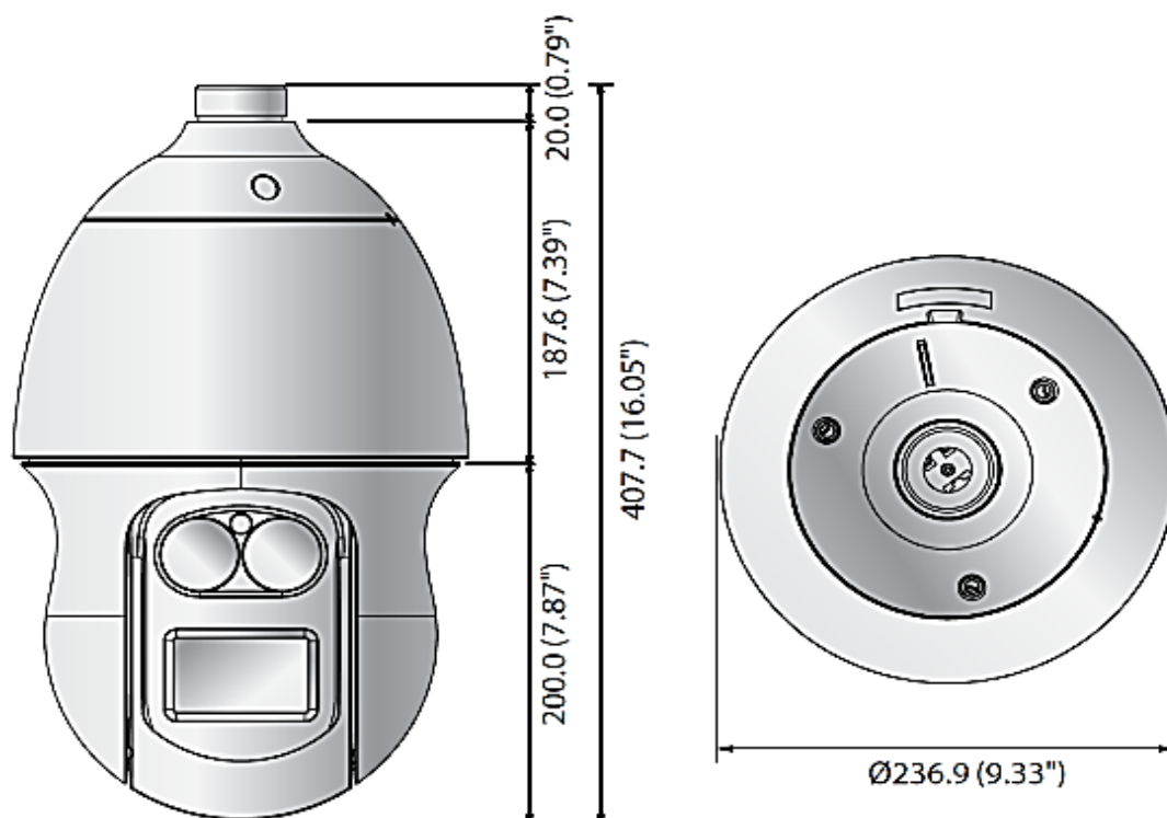
寸法図(mm)
