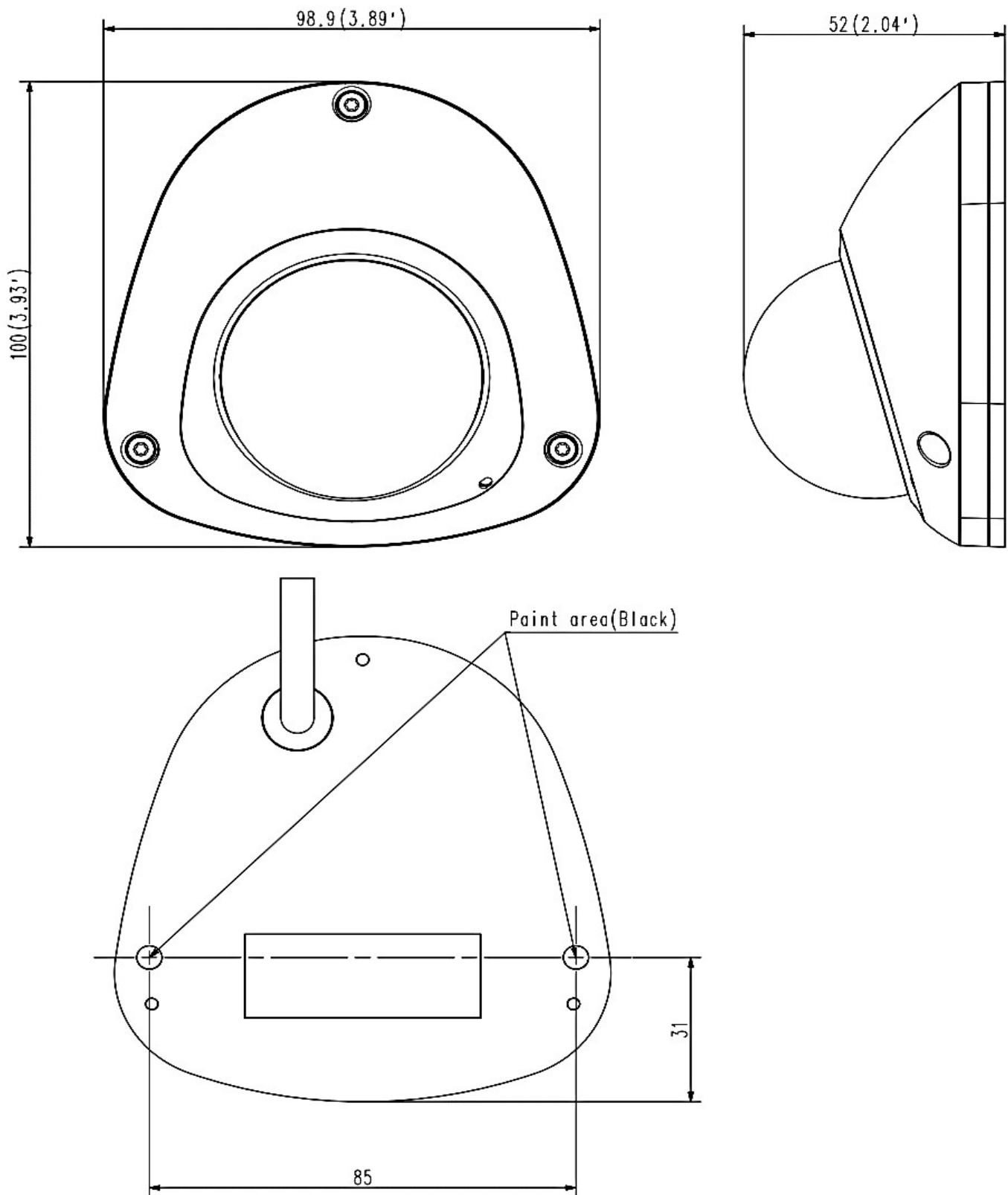
寸法図(mm)
