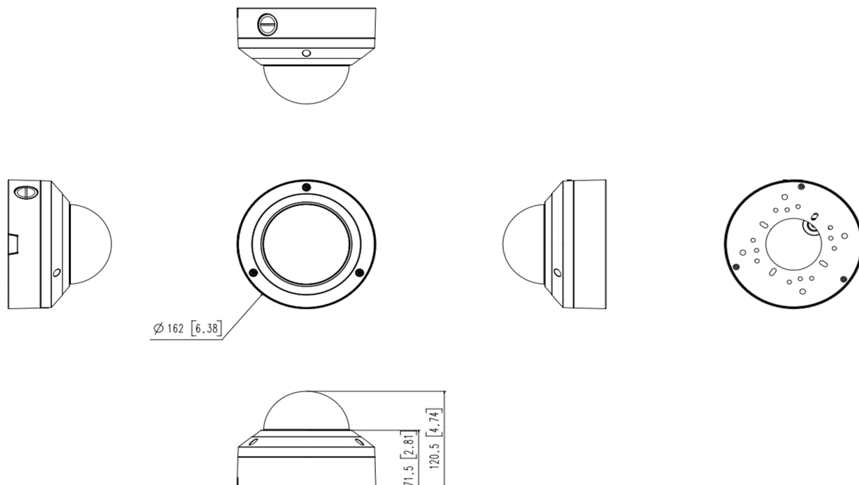
寸法図(mm)
