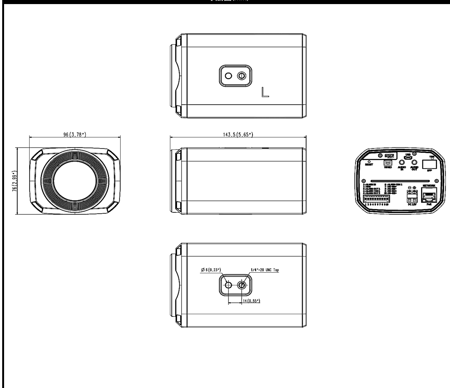
寸法図(mm)
