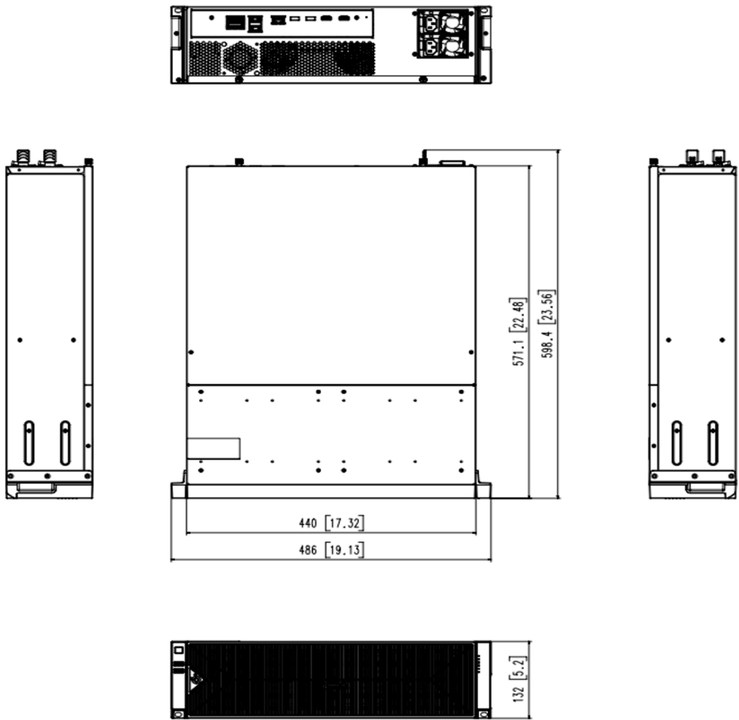
寸法図(mm)
