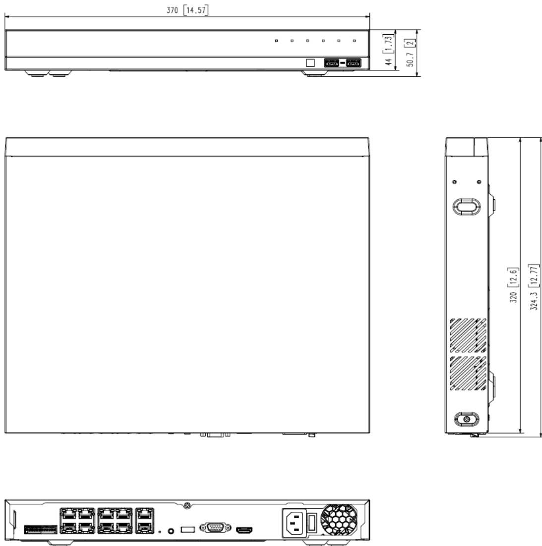
寸法図(mm)
