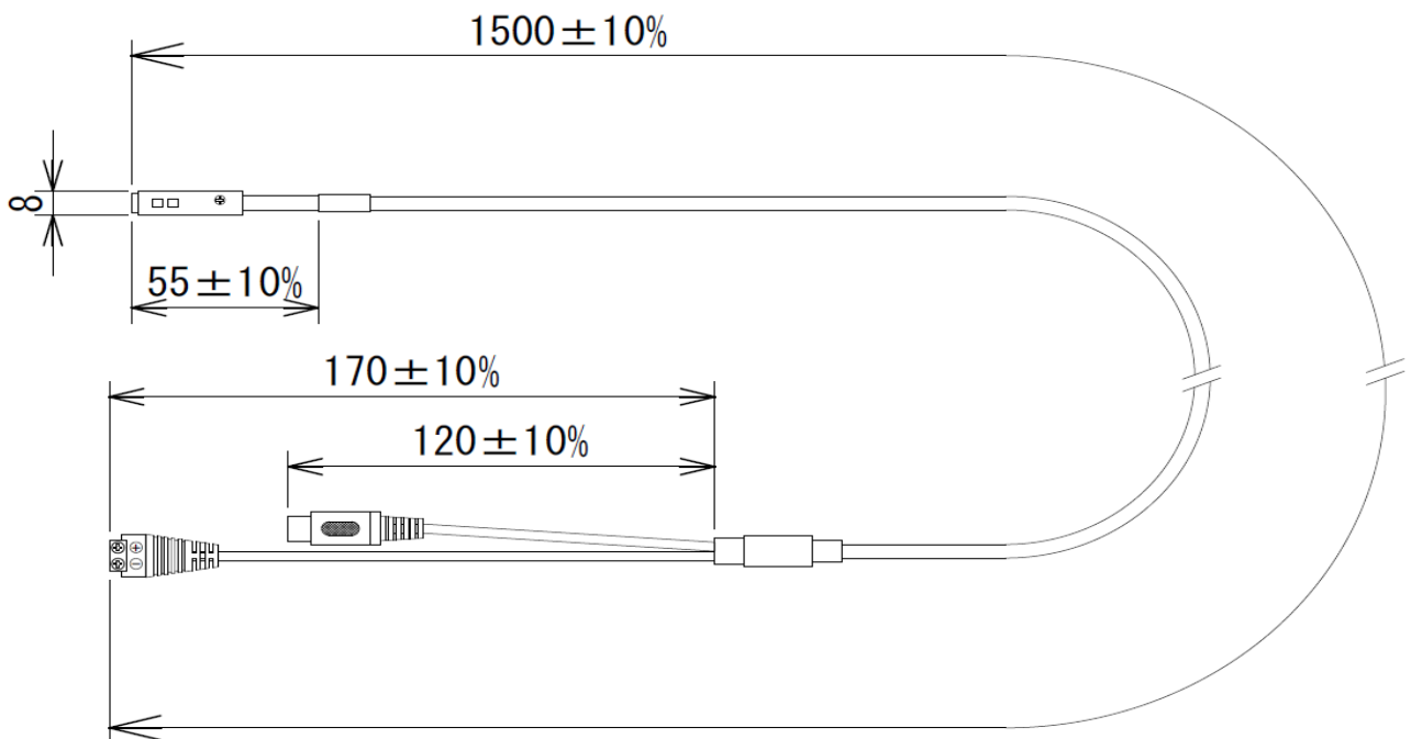
寸法図(mm)
