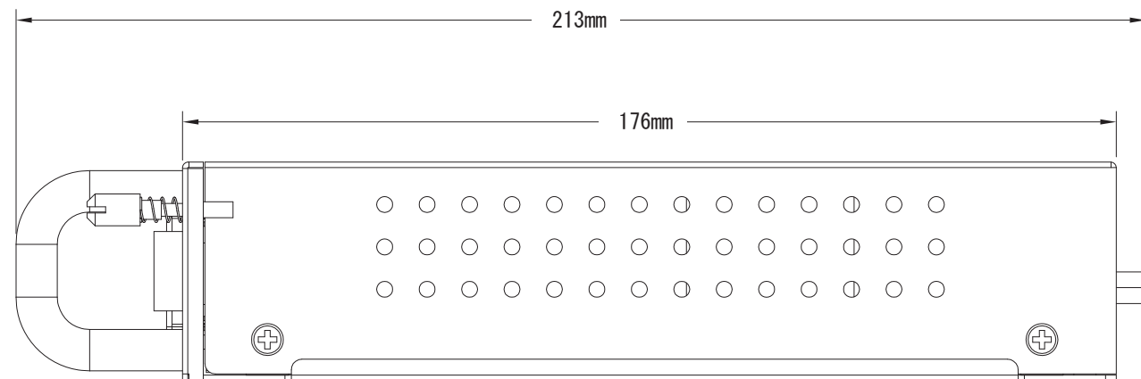
LEX1910-15外觀図
