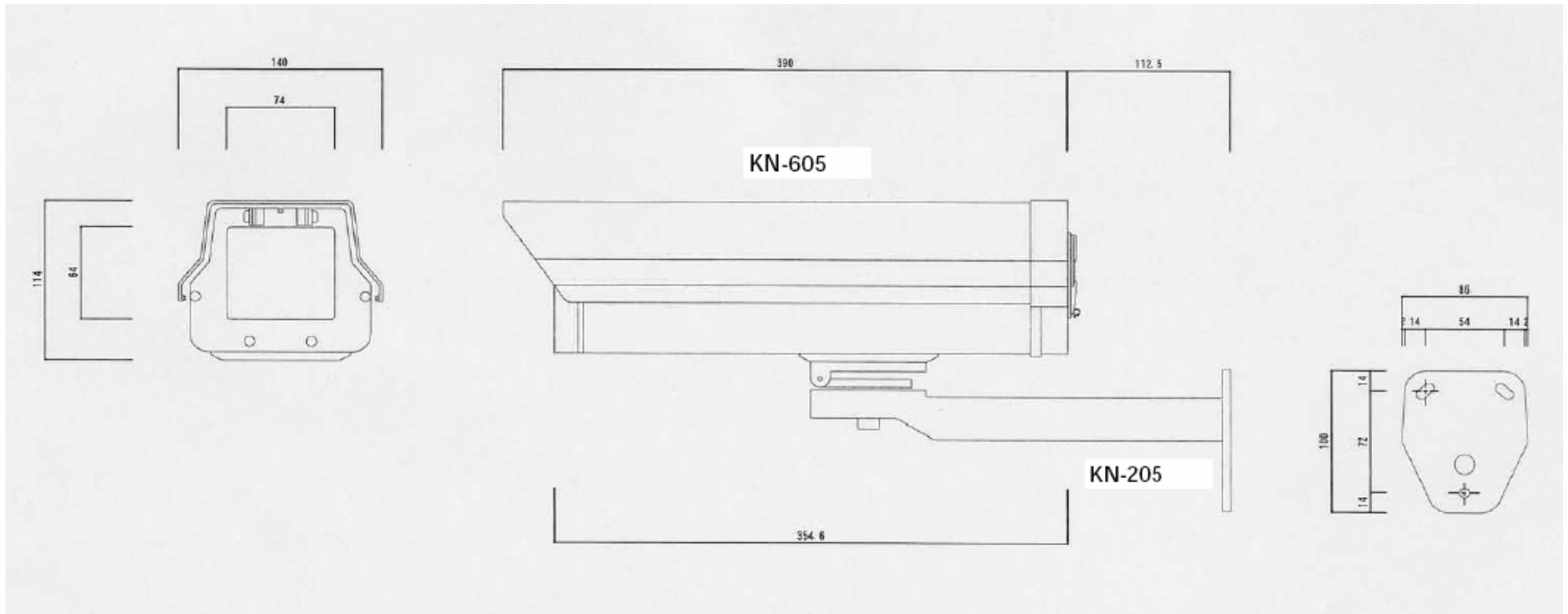
寸法図(mm)
