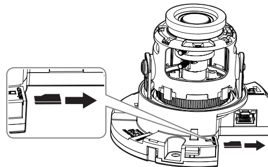
&lt;QND-6070R&gt;
