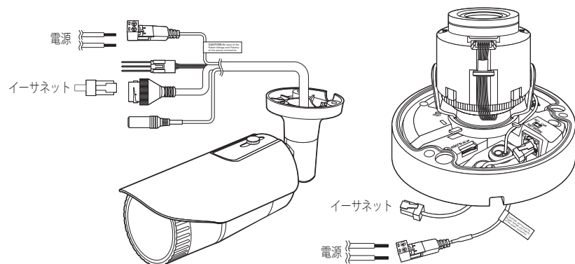
<QNO-6070R>
