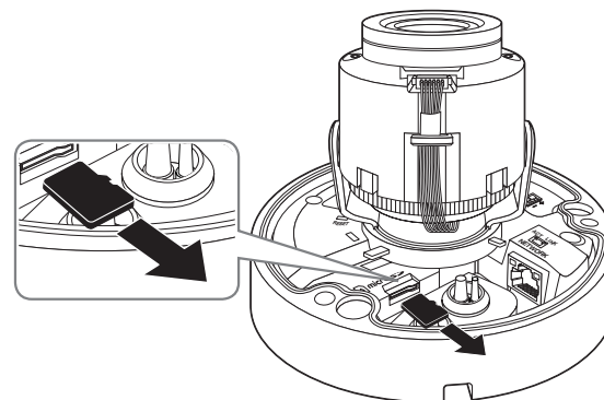
&lt;QNV-6070R&gt;
