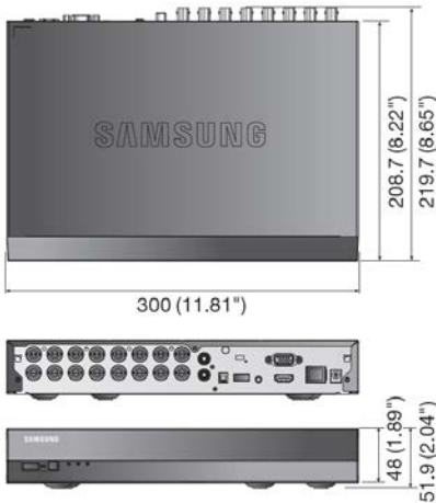
寸法(mm)
